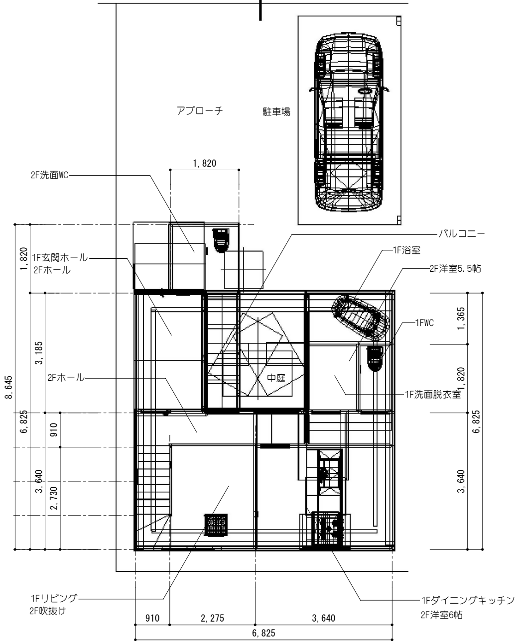
平面図 S=1/100
