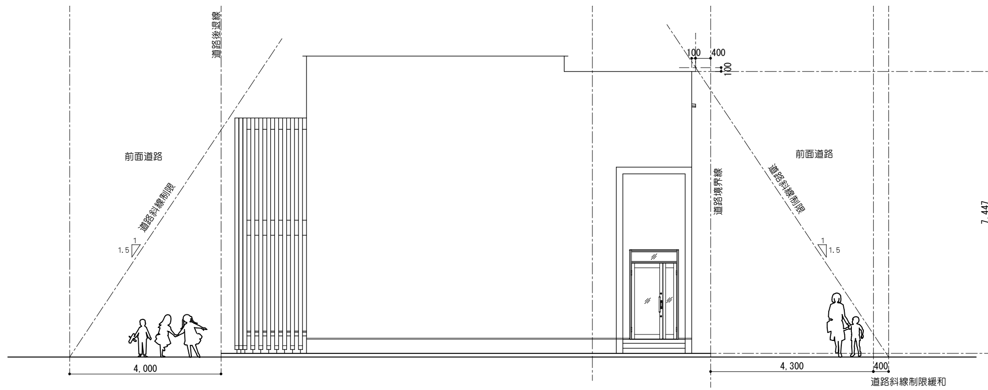
東側立面図 S=1/100 41-9-2
