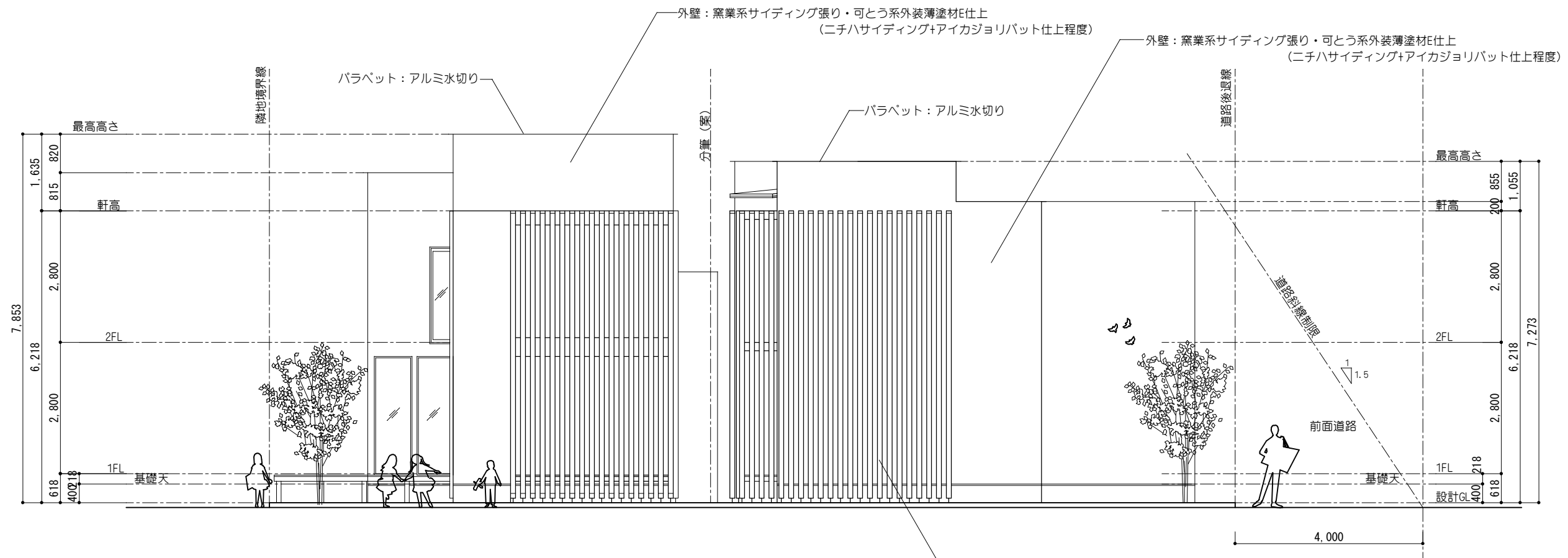
南側立面図 S=1/100
